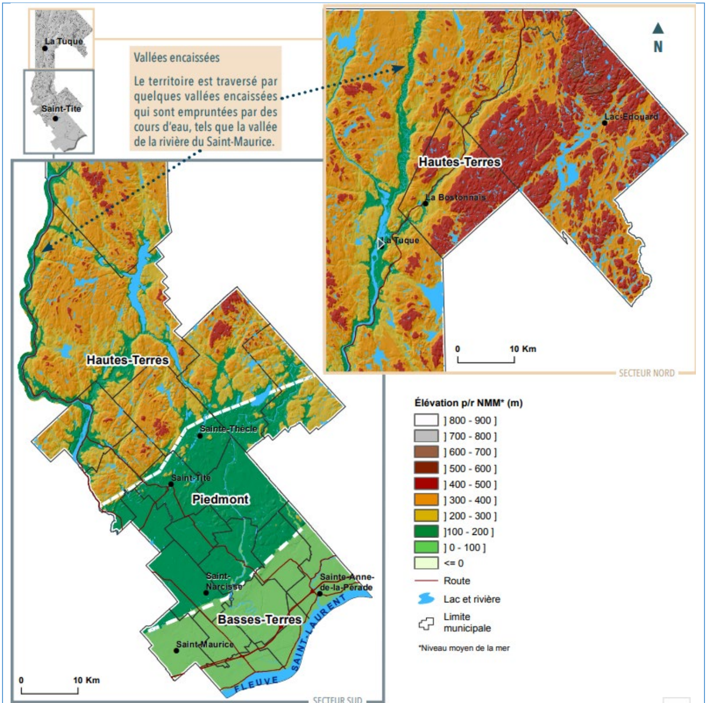
Figure 2 : Topographie de la zone d'étude de l'Atlas des connaissances sur les eaux souterraines de l'est de la Mauricie (CERM-PACES, 2022).
